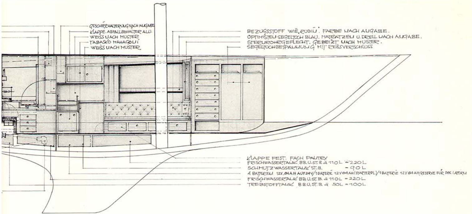
WANDANSICHT B. B. SEITE
