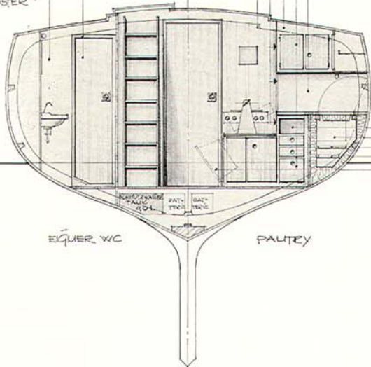
SPANT 6 VON VORNE GEGEHEN
