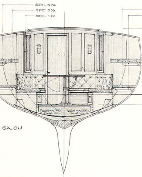
SPANT 5 VON ACHTERN GEGEHEN
